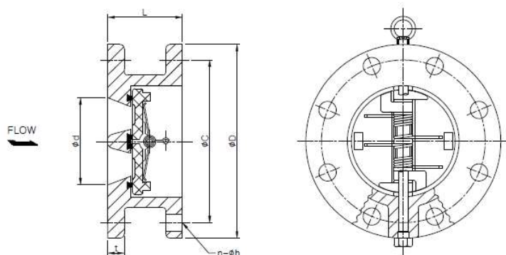
FLANGE
